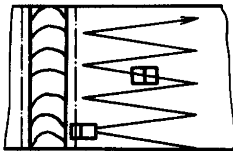
图 11 锯齿形扫查
