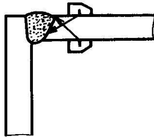
图 17 角接头
