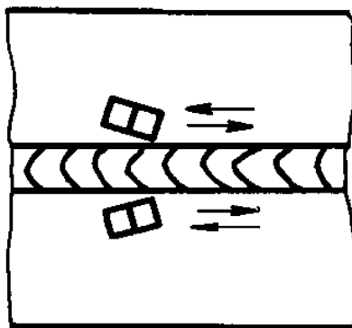
图 12 斜平行扫查
