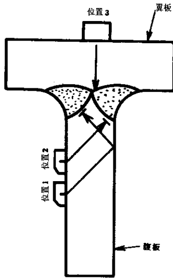
图 16 T型接头
